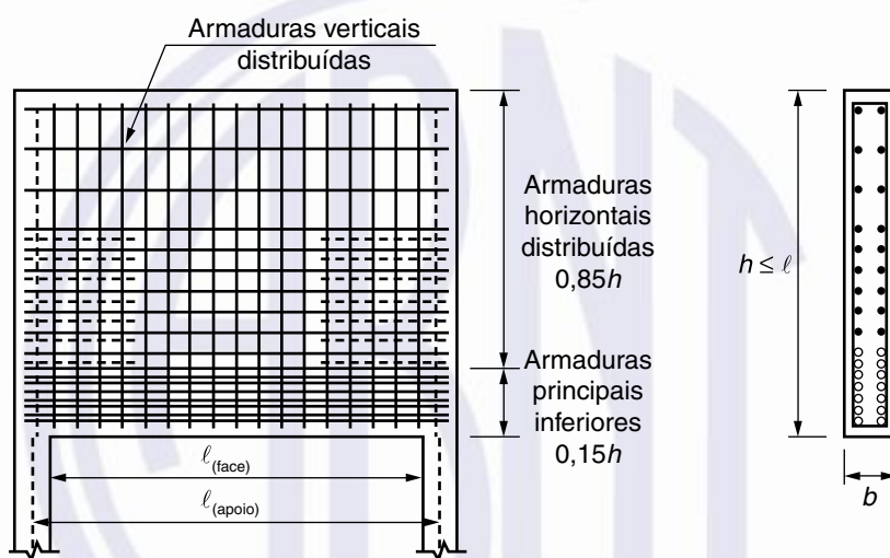
Figura 22.3 – Armação típica de viga-parede com h \leq \ell
