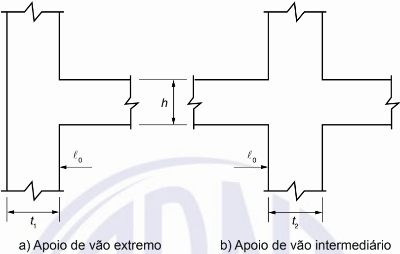
Figura 14.5 – Vão efetivo
