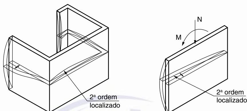
Figura 15.3 – Efeitos de 2ª ordem localizados
