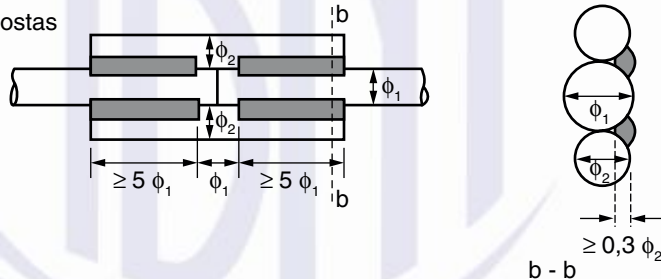
Figura 9.6 – Emendas por solda
